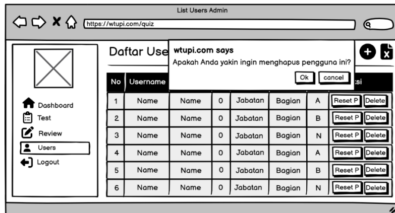
Gambar 3.41 Mockup Tombol Delete pada Menu Users Admin
