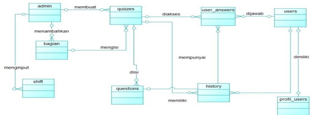
Gambar 3.17 Relasi Tabel CDM
