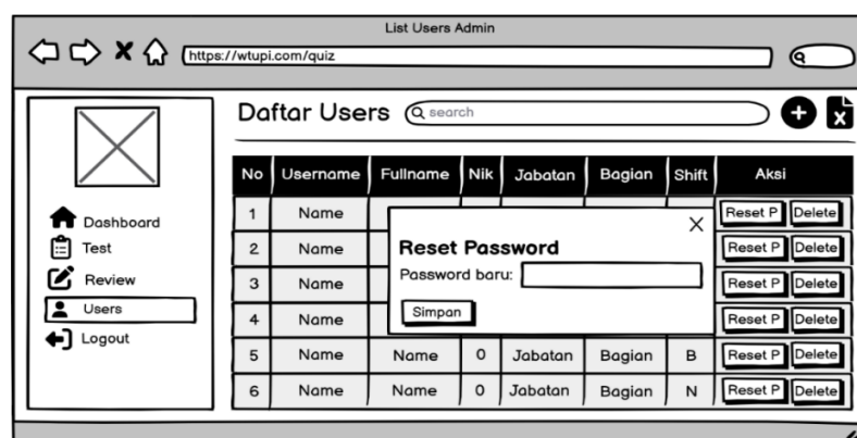
Gambar 3.40 Mockup Tombol Reset P pada Menu Users Admin
