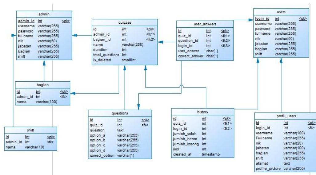
Gambar 3.19 Relasi Tabel PDM
