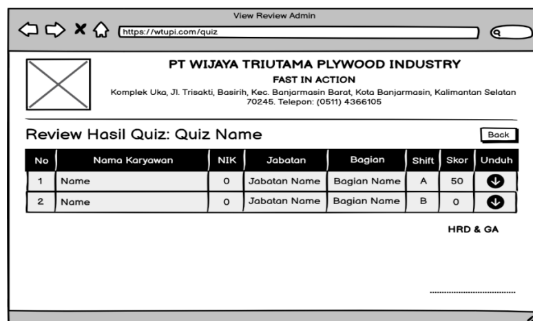
Gambar 3.35 Mockup Tombol View pada Menu Review Admin
