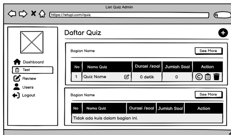
Gambar 3.24 Mockup Tombol See More pada Menu Test Admin
