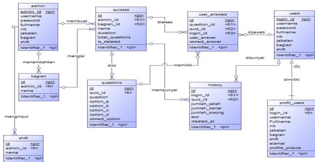
Gambar 3.18 Relasi Tabel LDM
